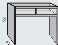
Toonbank MX-28 € 490,00 br 115 x d 60 x h 92cm Kleur afgebeeld: Zilver/ Wengé
